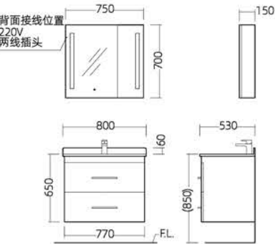
安装尺寸图
