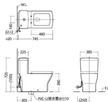
安装尺寸图
