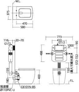
安装尺寸图
