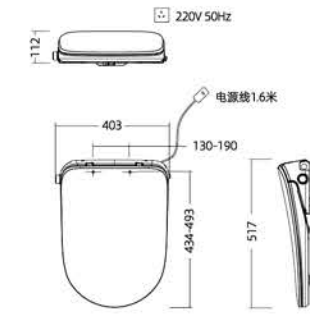
安装尺寸图
