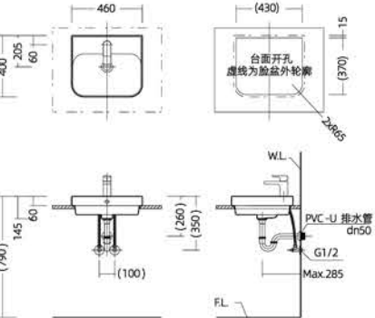
安装尺寸图
