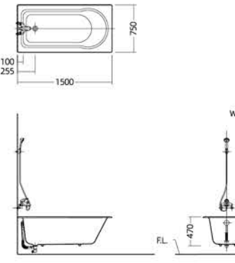
安装尺寸图
