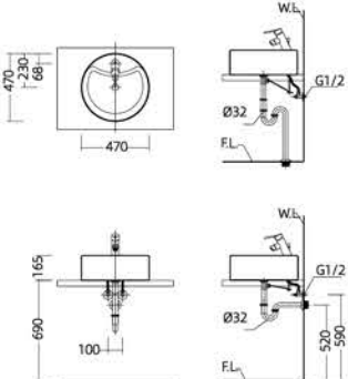
安装尺寸图
