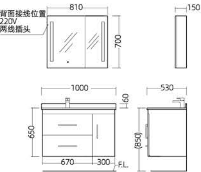
安装尺寸图
