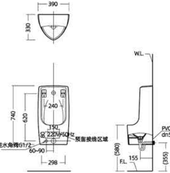
安装尺寸图
