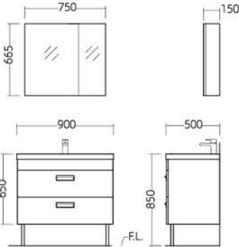
安装尺寸图
