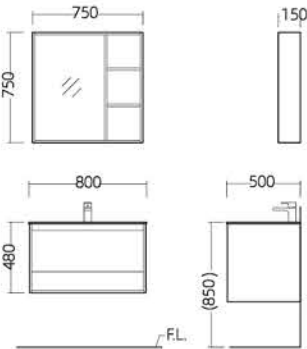
安装尺寸图
