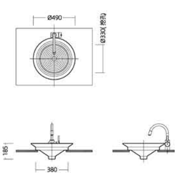
安装尺寸图
