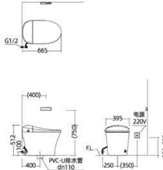
安装尺寸图
