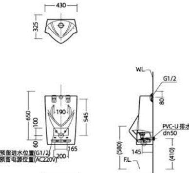
安装尺寸图
