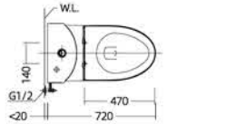
安装尺寸图
