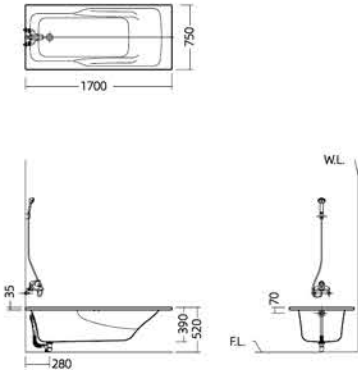
安装尺寸图
