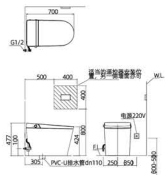
安装尺寸图
