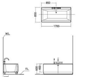
安装尺寸图
