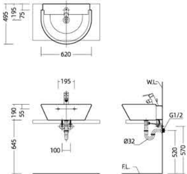
安装尺寸图
