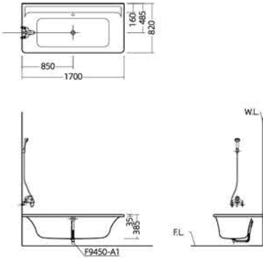
安装尺寸图
