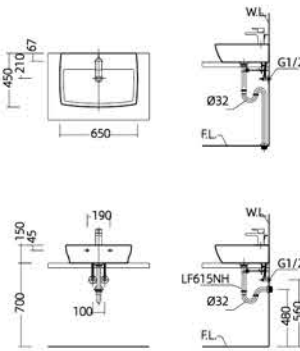
安装尺寸图
