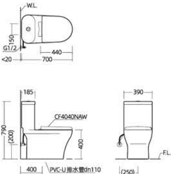
安装尺寸图
