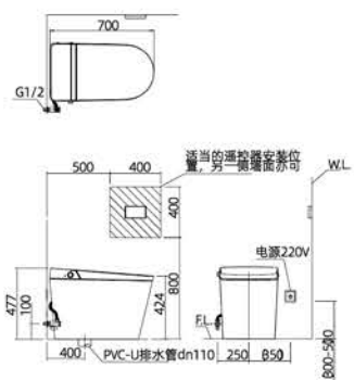
安装尺寸图
