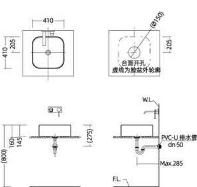
安装尺寸图
