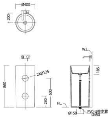
安装尺寸图
