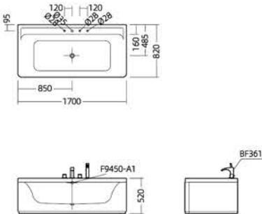
安装尺寸图
