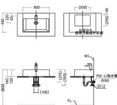
安装尺寸图
