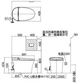
安装尺寸图
