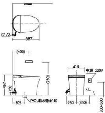
安装尺寸图
