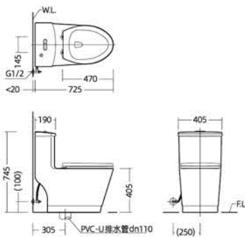
安装尺寸图
