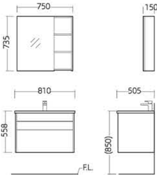
安装尺寸图
