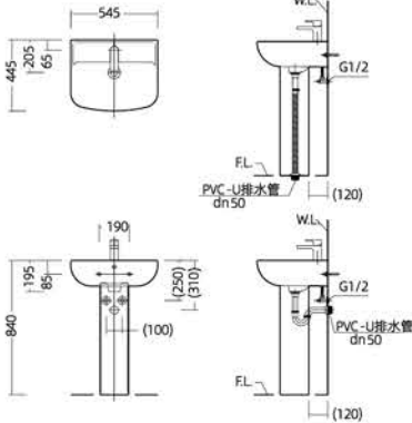
安装尺寸图
