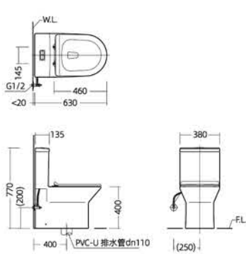
安装尺寸图
