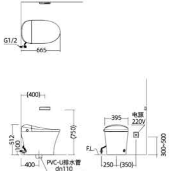
安装尺寸图
