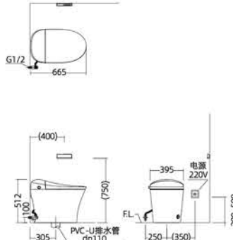
安装尺寸图
