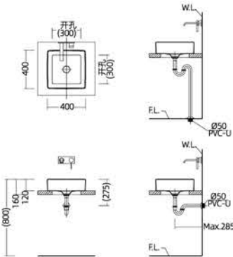
安装尺寸图
