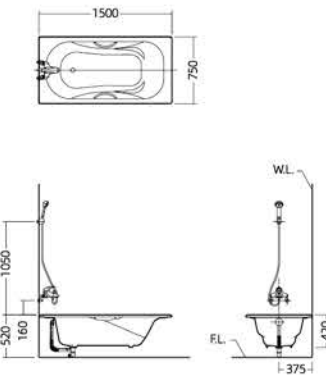
安装尺寸图
