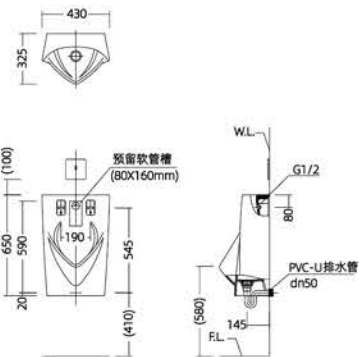
安装尺寸图
