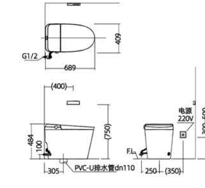
安装尺寸图
