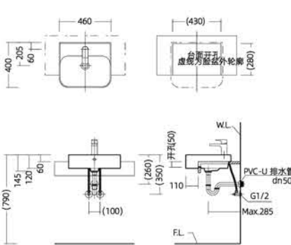
安装尺寸图
