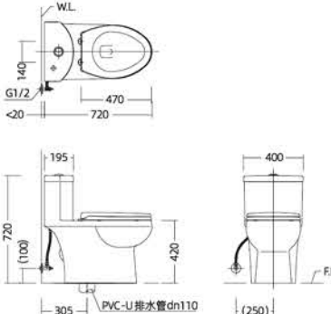
安装尺寸图
