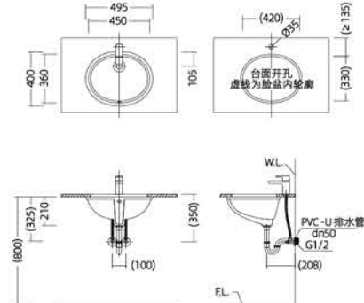
安装尺寸图
