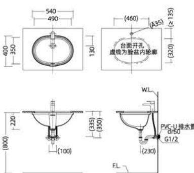
安装尺寸图
