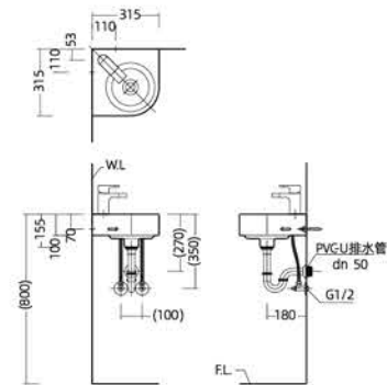
安装尺寸图
