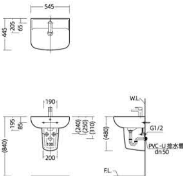
安装尺寸图
