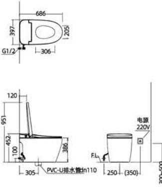
安装尺寸图
