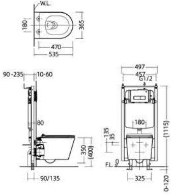
安装尺寸图
