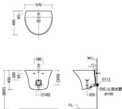
安装尺寸图
