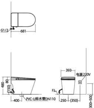
安装尺寸图
