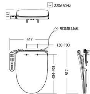
安装尺寸图
