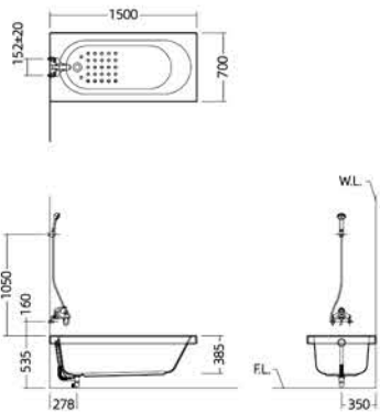
安装尺寸图
