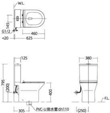
安装尺寸图
