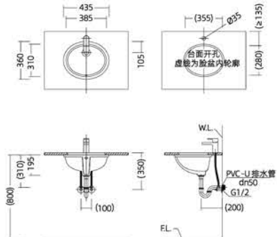
安装尺寸图
