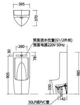
安装尺寸图
