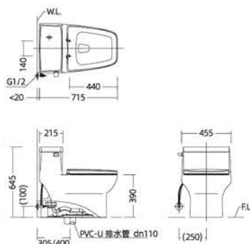
安装尺寸图
