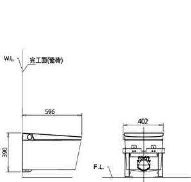
安装尺寸图
