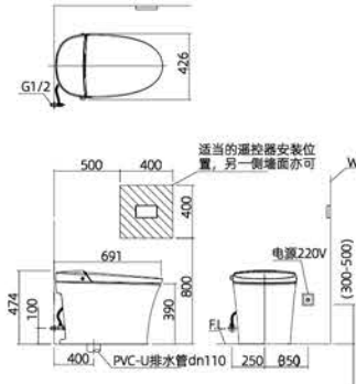
安装尺寸图
